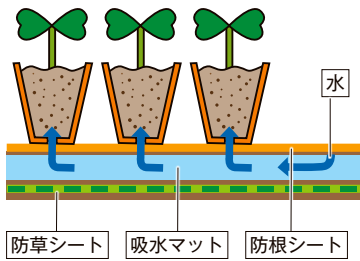
水は吸水マットを伝わって、セルトレイ底面から吸われる
